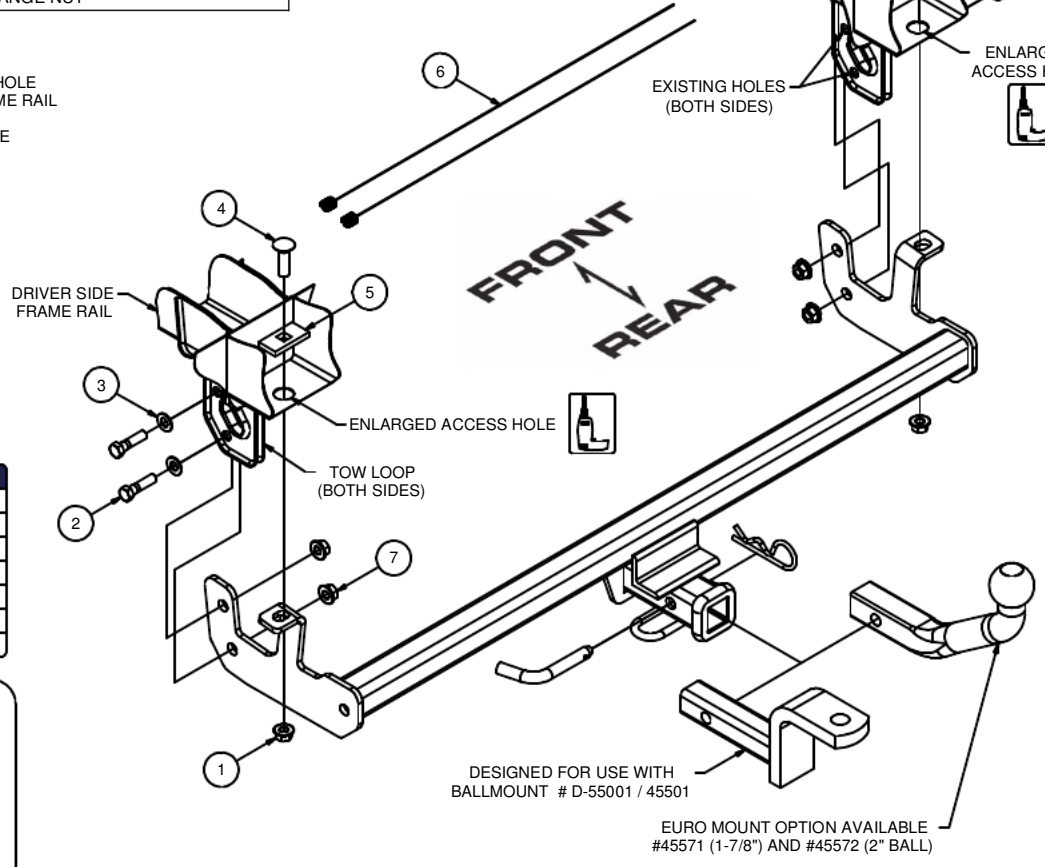
HOLE ENLARGEMENT DIAGRAM
